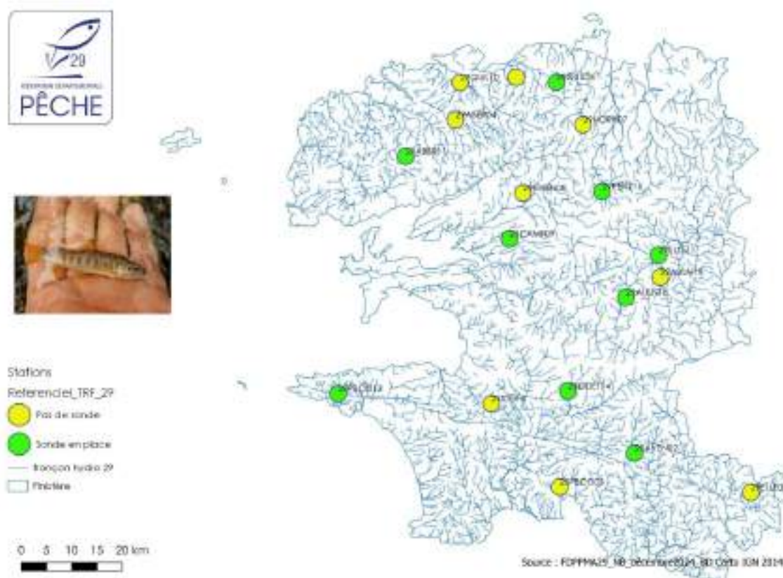
Carte n°4 : Localisation des stations « Température »_2024
